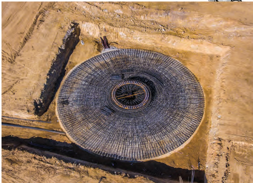
Πλατεία και θεμέλιο Α/Γ KR-03
